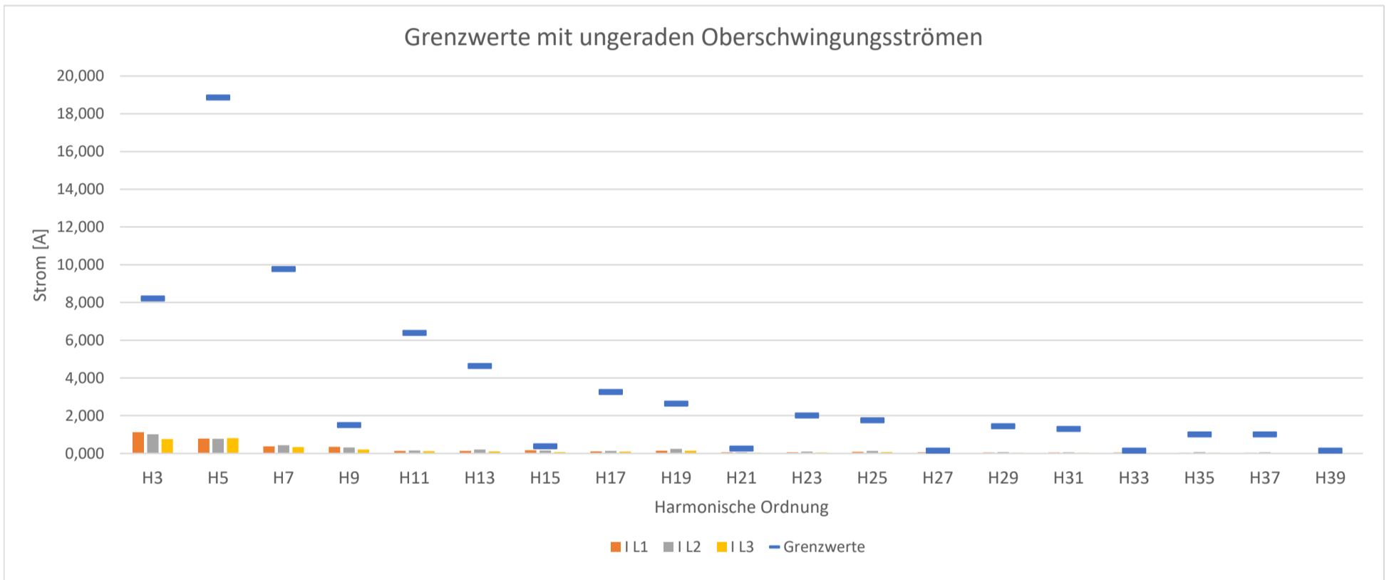
Grenzwerte mit Oberschwingungsströmen (ungerade Harm., alle Phasen):
