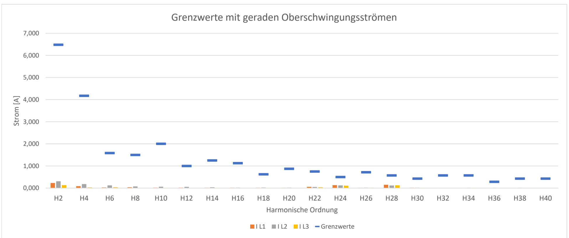
Grenzwerte mit Oberschwingungsströmen (gerade Harm., alle Phasen):
