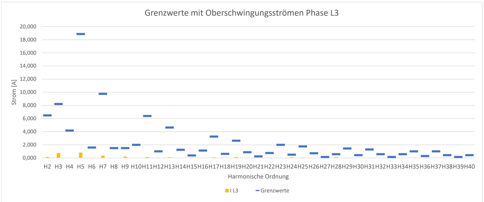
Grenzwerte mit Oberschwingungsströmen (alle Harm., Phase L3):
